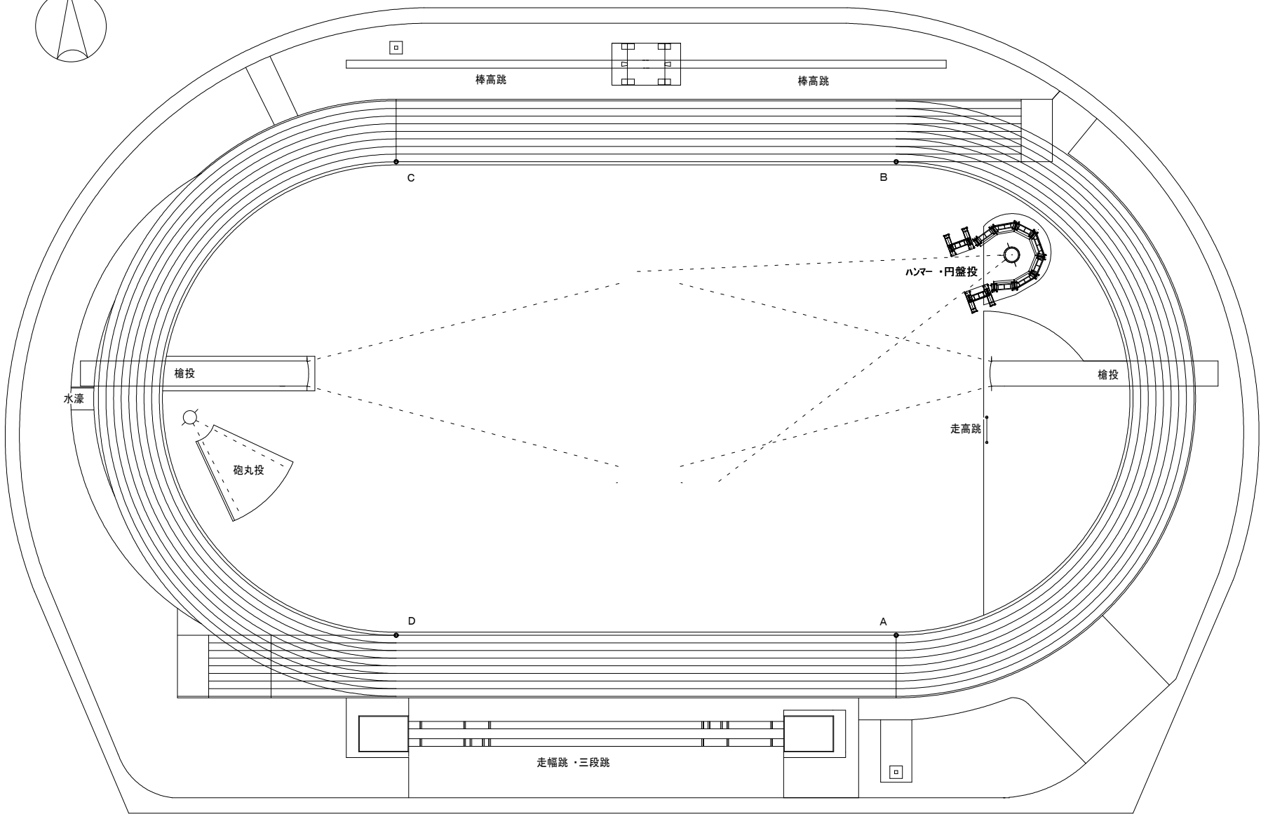
秋留台公園陸上競技場 S=1 : 600
